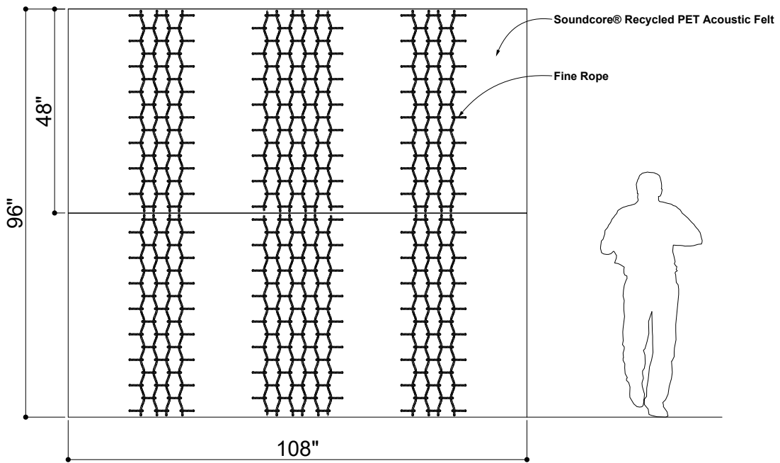
② ELEVATION 2
